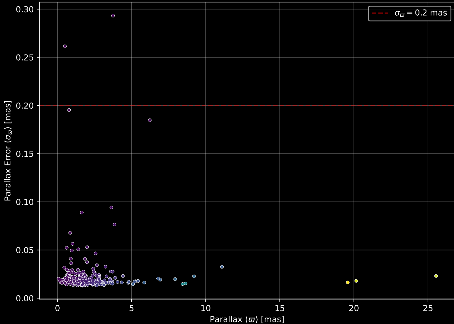
GALAH DR4 Field: [7028] Parallax Quality (n= 290)
