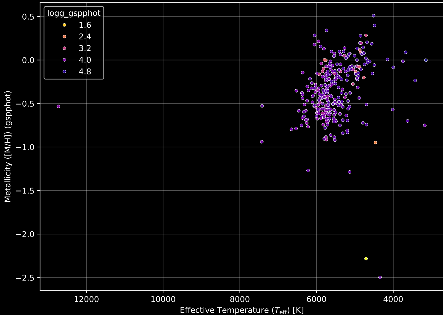
GALAH DR4 Field: [7028] Stellar Population Parameters (n= 290)
