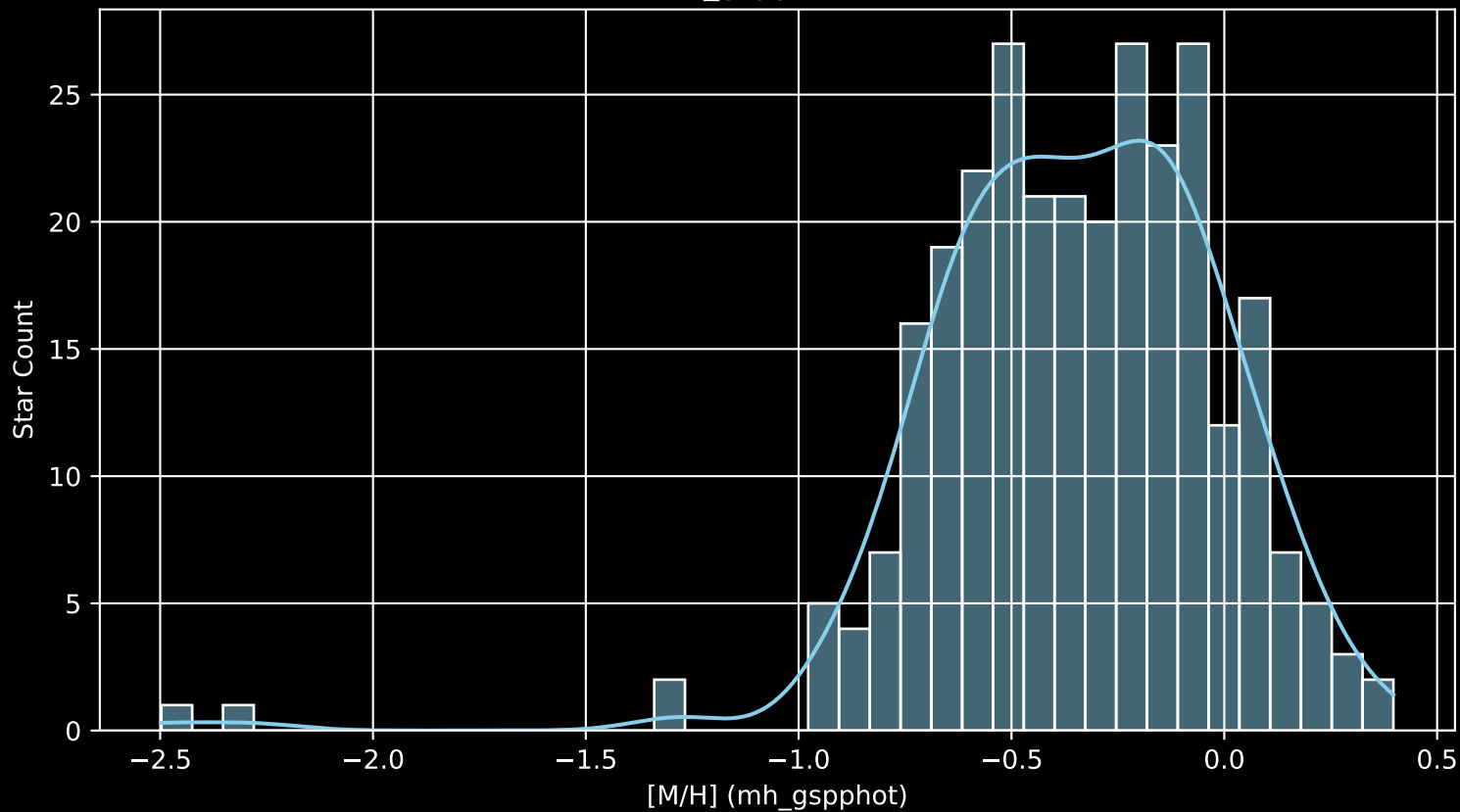
GALAH DR4 Field: [7028] [M/H] (mh_gspphot) (n= 289)
